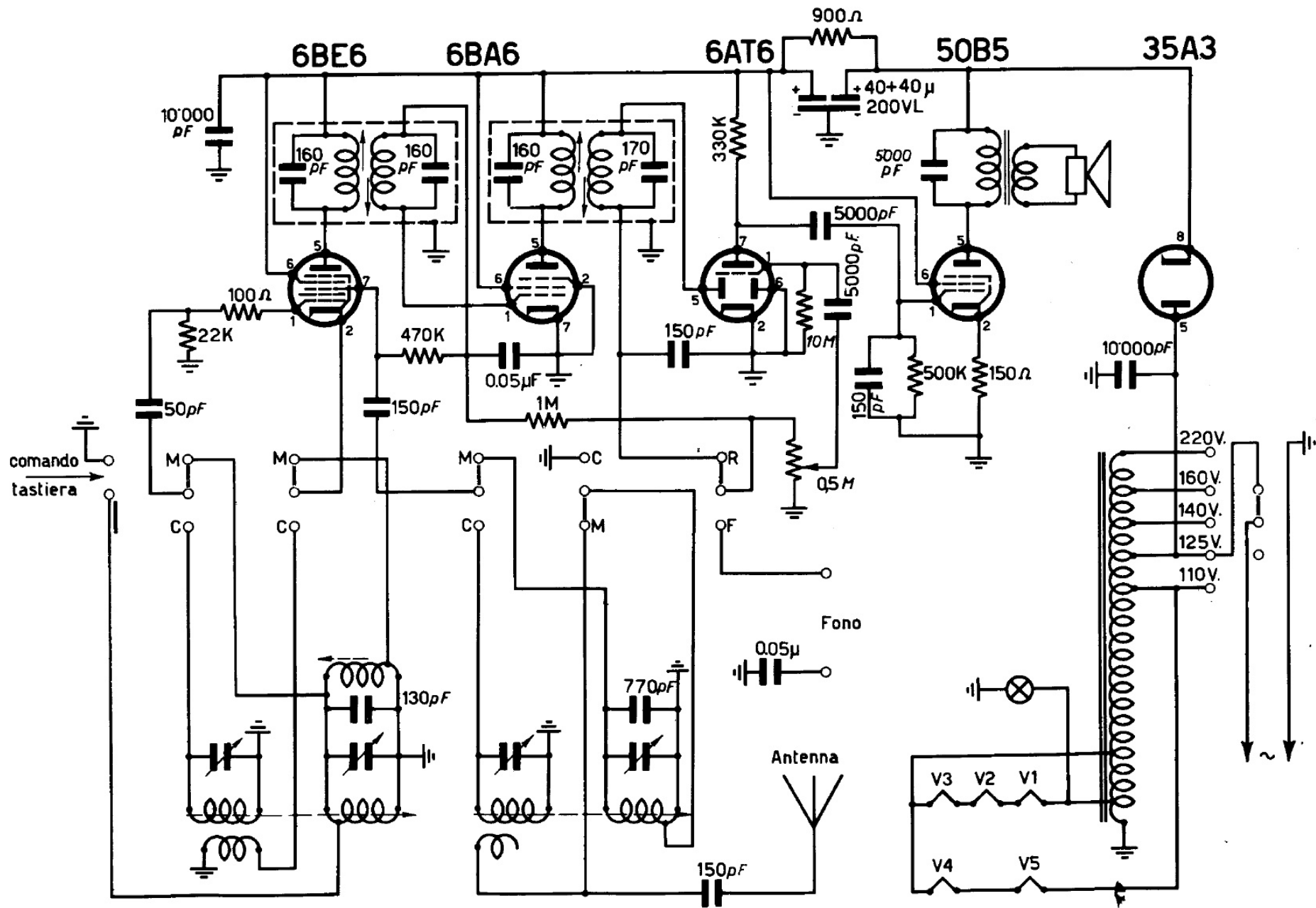
SCHEMA ELETTRICO DEI RADIORICEVITORI G.B.C. AR/4 e AR/5
